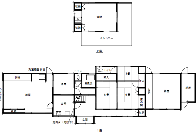
間取り図
