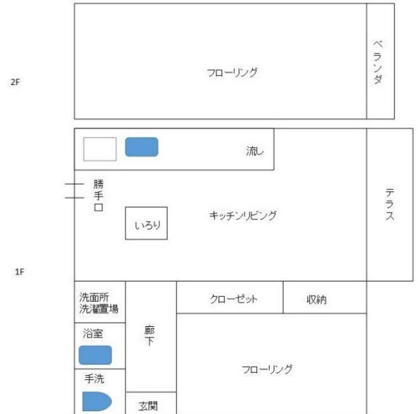
間取り図
